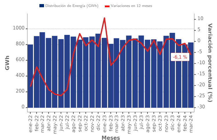
■ Evolución Distribución de Energía, región de Antofagasta (enero 2022 - marzo 2024)
